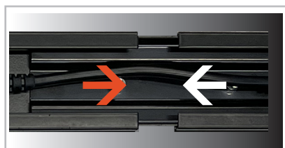
Узел соединения светильника PSO-02 L со светильником PSO-02 (вид с обратной стороны)
