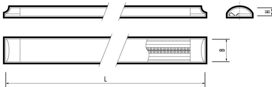
Рис. №1 Светильник PPO-03
