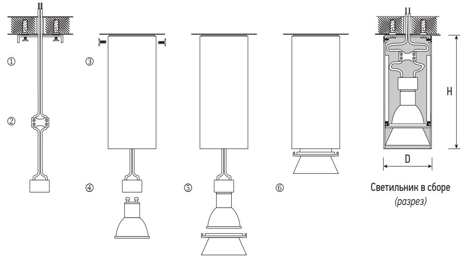
Рис. №1 Схема подключения светильника PDL-R/PDL-S
