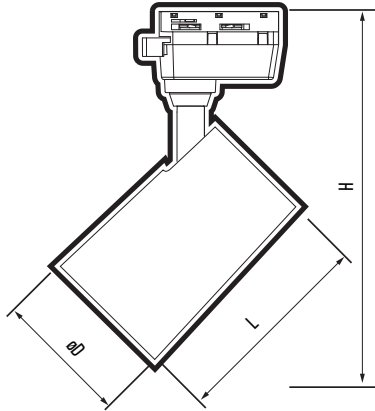
Рис 1. Прожектор PTR 07
