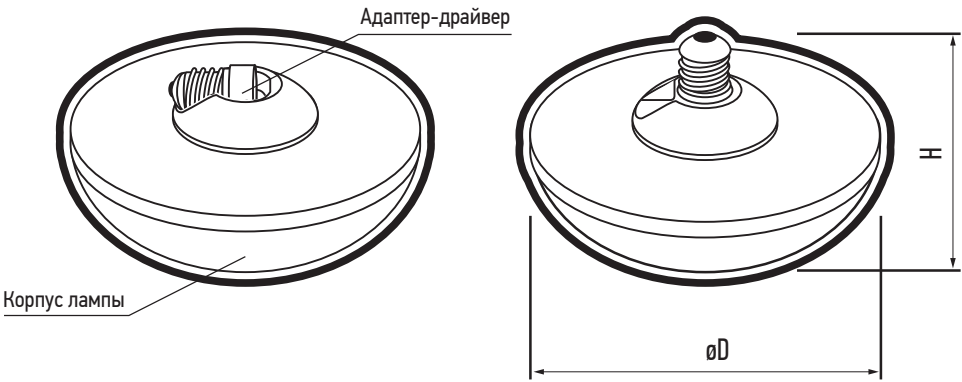
Рис.1 PLED-HP-UFO 55w в транспортном положении
