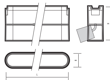
Рис. 1 MTR16 11R FROST 90°
