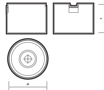
Рис. 2 MTR16 32
