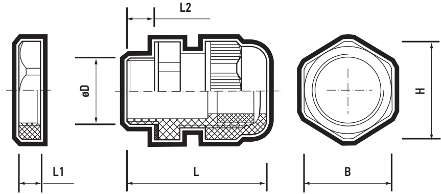
Рис. 1 Сальник PCG
