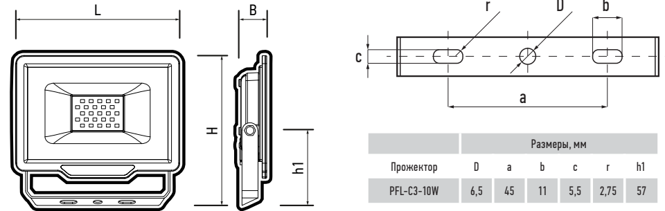
Рис. 1 Прожектор PFL-C3
