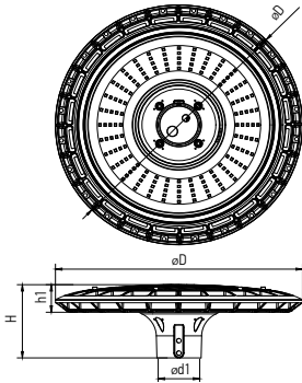
Рис.1 Светильник PGL 04
