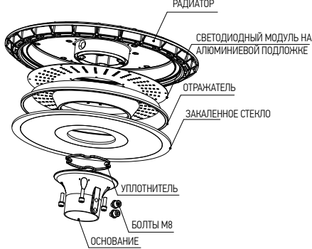
Рис.2 Взрыв-схема светильника PGL 04
