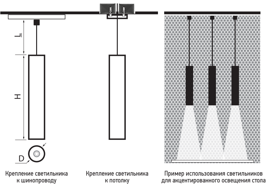
Рис.1 Прожектор PTR 2310
