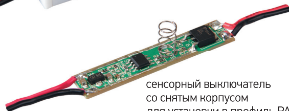
сенсорный выключатель
