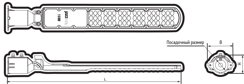
Рис.1 Светильник консольный светодиодный серии PSL 09
