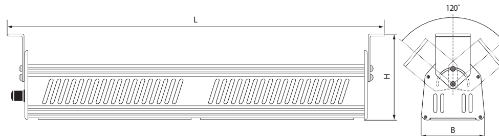
Рис. 1 Светильник PPI-01
