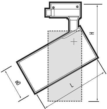
Рис.1 Прожектор PTR 0724 Agro White
