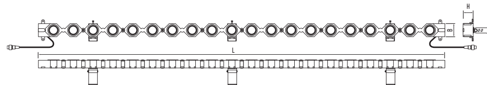
Рис.1 Светильник PWW 1000 24V. Габаритные размеры
