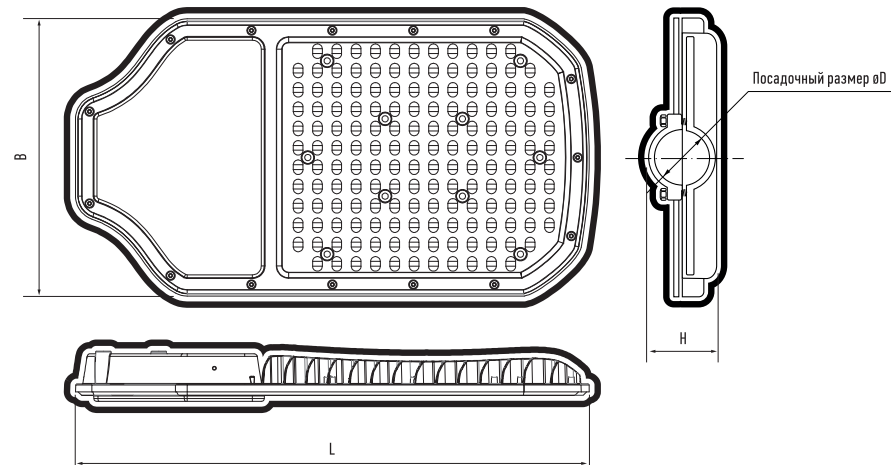
Рис.1 Светильник PSL 05-2
